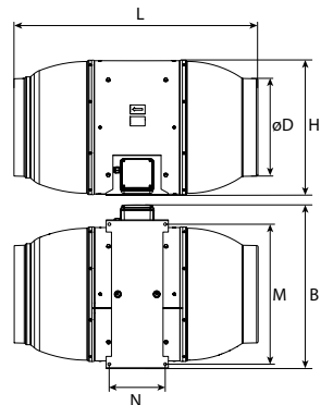
TT Silent-M 200/250/315
